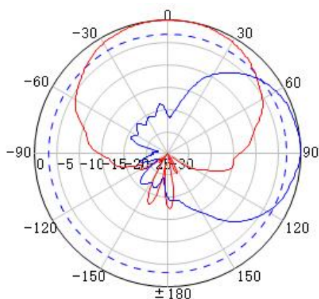
方向图
