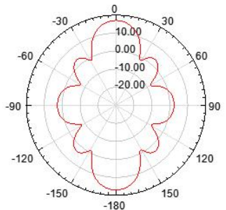
3.9G 水平面方向图
