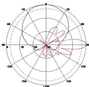
方向图
