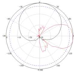
5GHz 频段方向图
