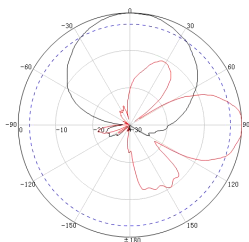
1.6G&2.4GHz 频段方向图
