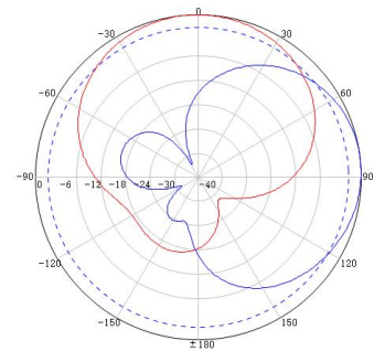
典型方向图 2.4GHz
