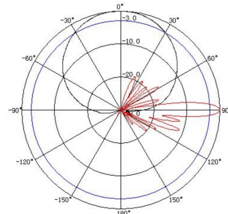
3300-3800MHz 频段方向图
