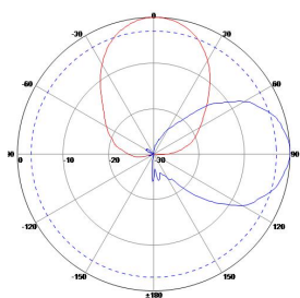
辐射方向图
