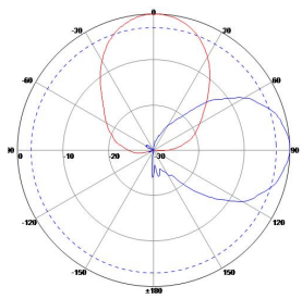
辐射方向图
