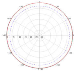
水平面方向图
