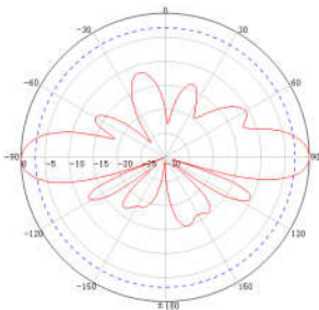
垂直面方向图
