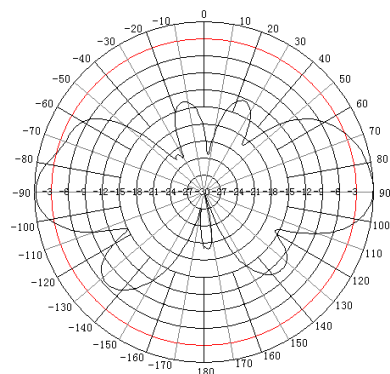
3.5GHz E面
