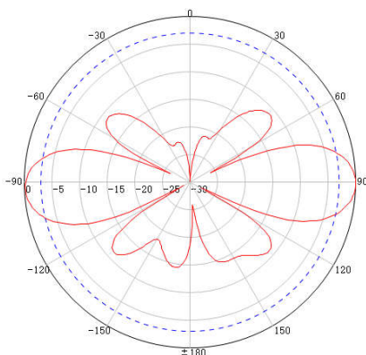
垂直面方向图
